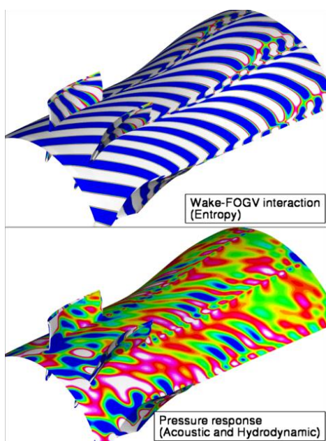
Fan-OGV interaction
